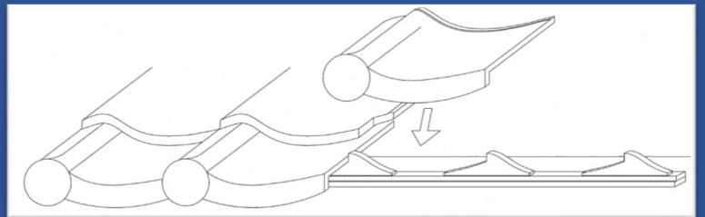
設置施工例
